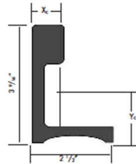
Type IV Rib
