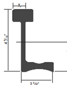
Type VI Rib
